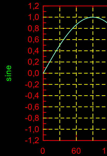
PLplot
